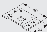
4972 Krokbeslag
