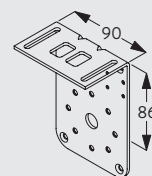
4904 Fäste (131 mm)
