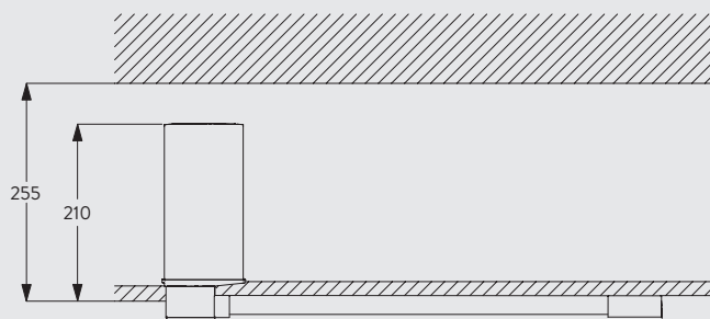
Montering med beslag 3004 i tak
