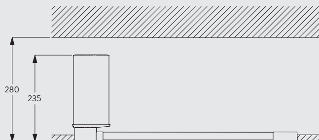
Montering med profil 10862 infälld i tak
