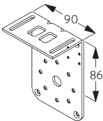
SG 4904 Bracket (set SG 4949)
